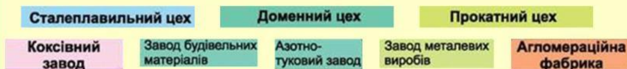
Схема металургійного комбінату повного циклу
