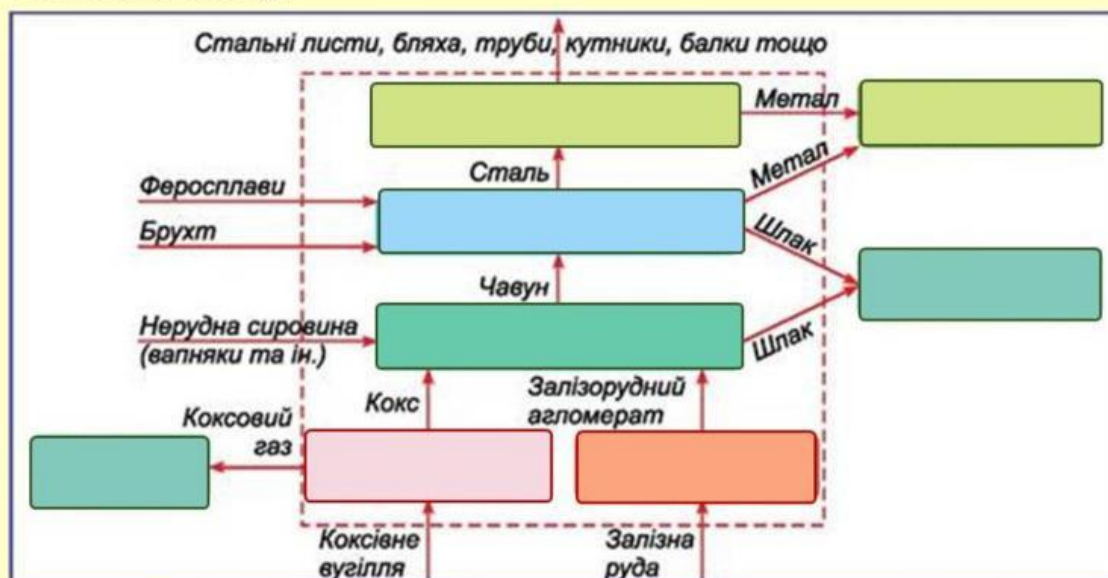
Схема металургійного комбінату повного циклу
