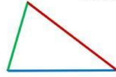
TRIÁNGULO ISÓSCELES
