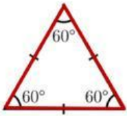
TRIÁNGULO EQUILÁTERO
