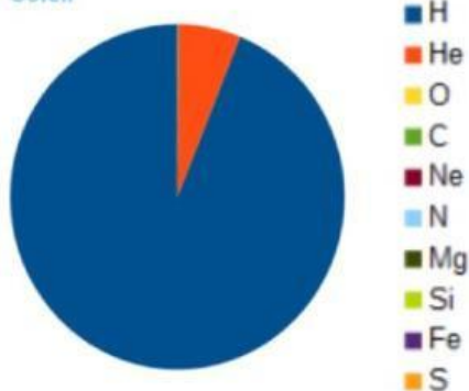
Composition du soleil
