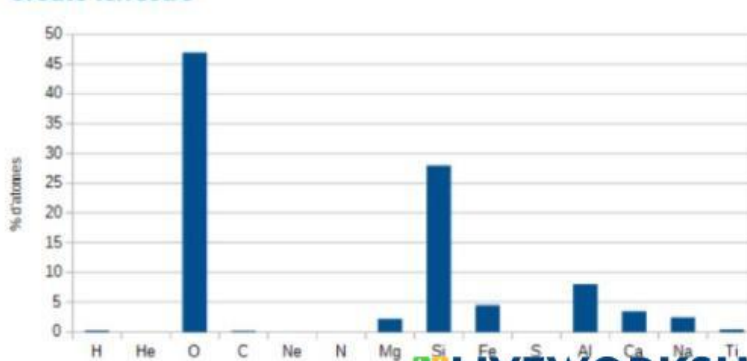
Composition de la croûte terrestre
