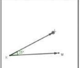
Ilustrasi Geometri dan Besar Sudut
