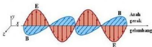
Gambar 9. Vektor perubahan medan listrik tegak lurus vektor perubahan medan magnet
