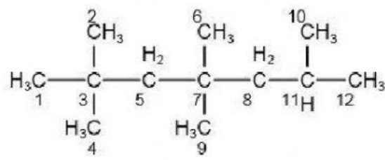
(Senyawa 2)
