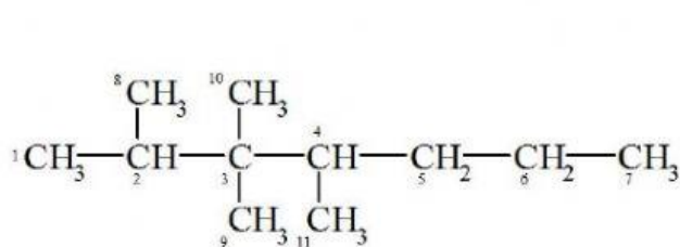
(Senyawa 1)
