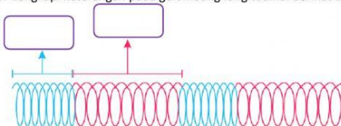
Gelombang Longitudinal
