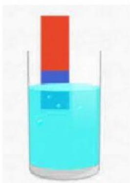
Na 2 CO 3
