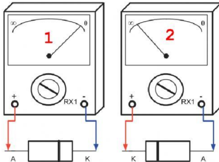
รูปที่ 1.1 การตรวจสอบ Diode
