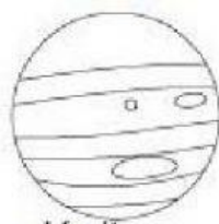
Júpiter
