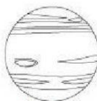
Netuno
