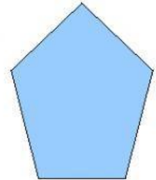
pentàgons
