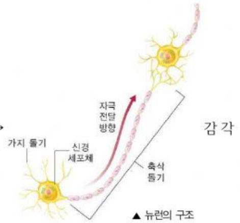
▲ 뉴런의 구조
