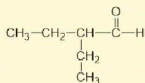
2-etilbutanal
