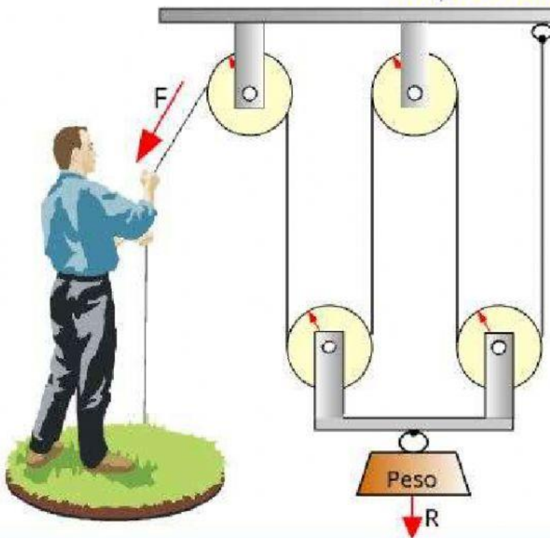
Polipasto doble
