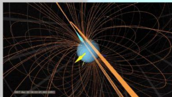
Campos magnéticos
