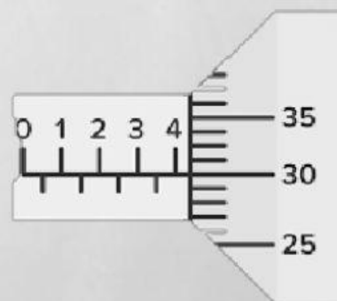
Mikrometer Sekrup
