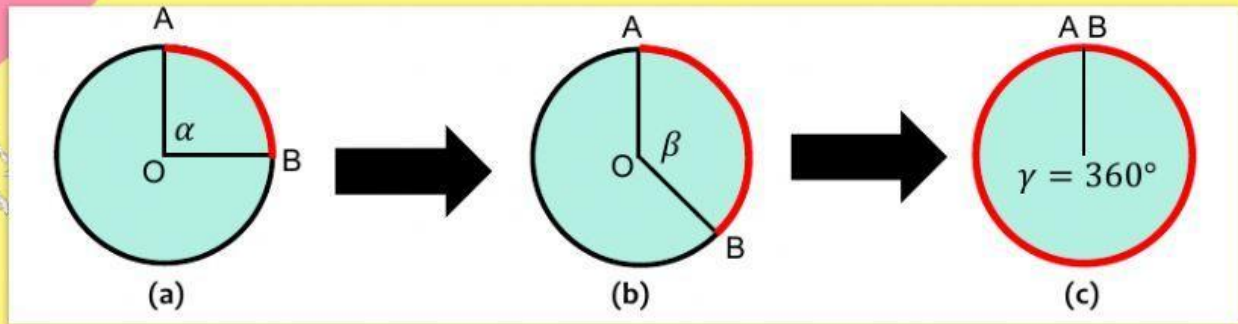
Gambar 18. Hubungan Sudut Pusat dan Panjang Busur
