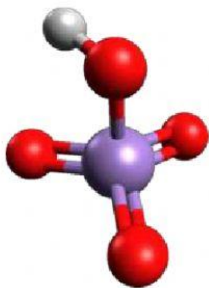
7. \text{HMnO}_4
