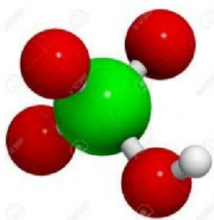
6. \text{HClO}_4
