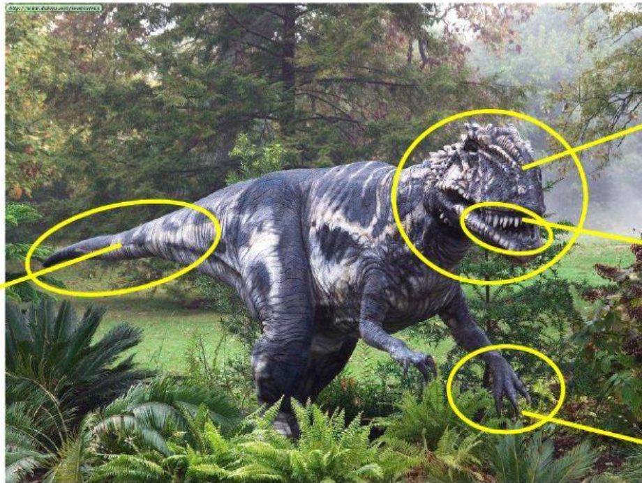
Le mégalosaure
