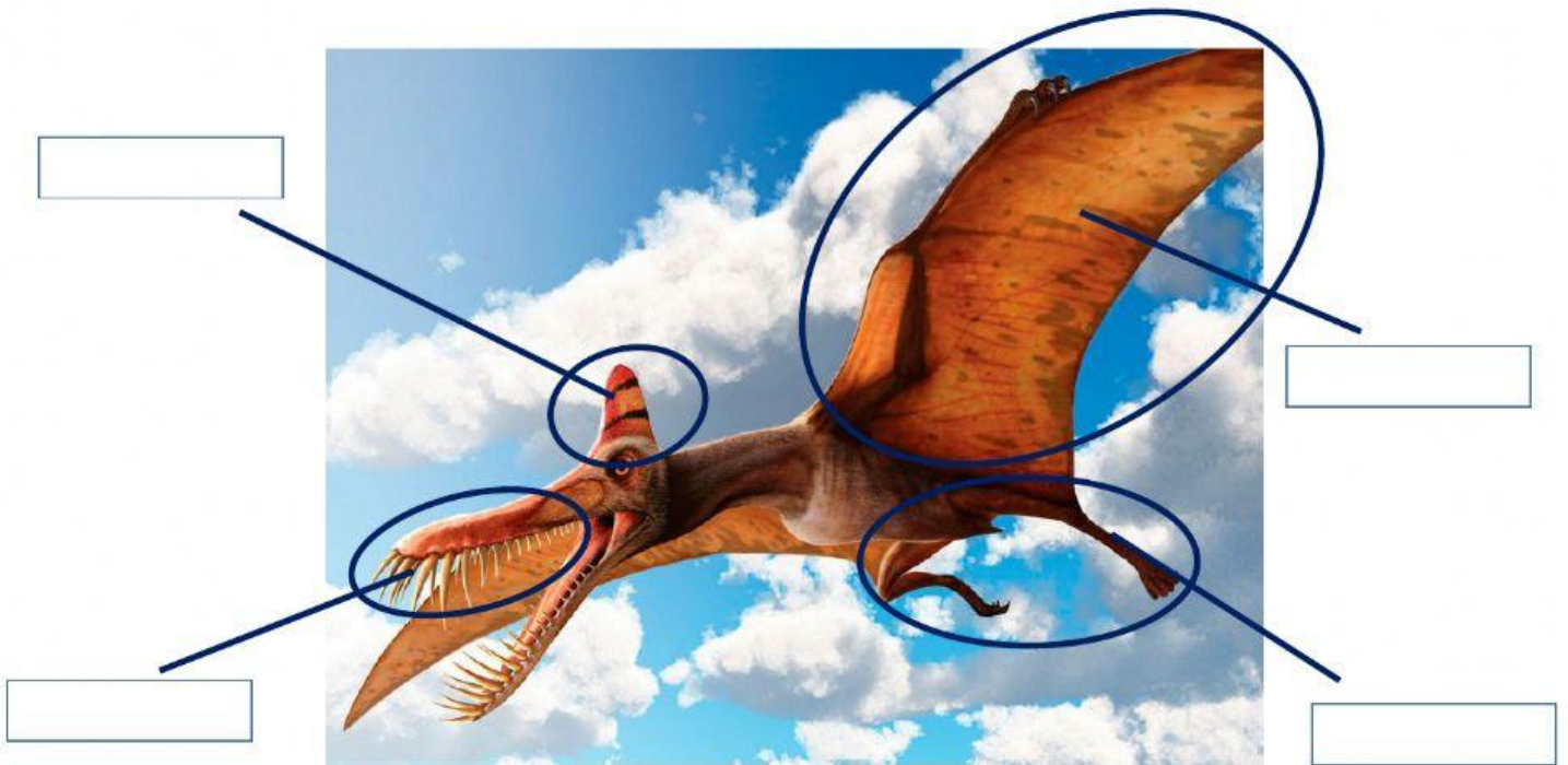
Le ptérodactyle
