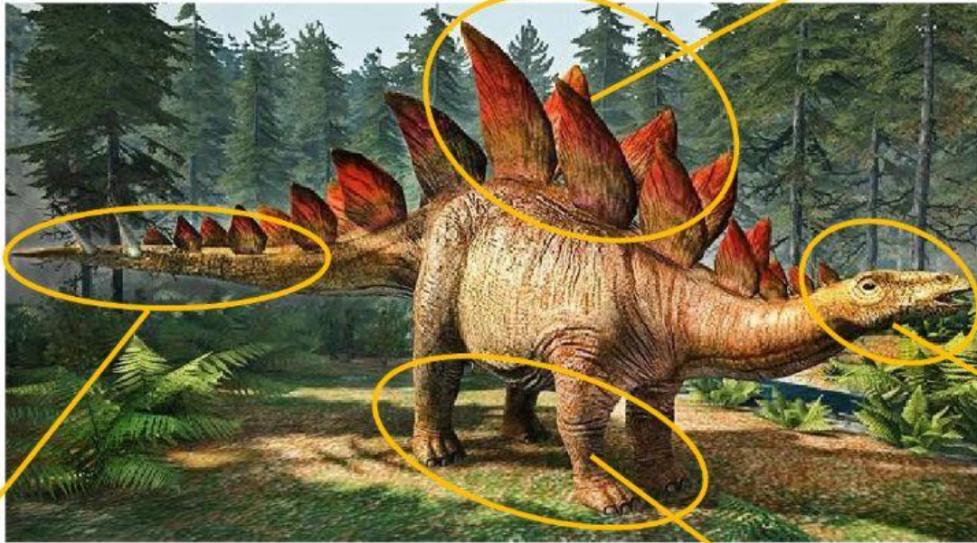
Le stégosaure
