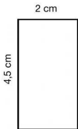
paral·lelogram (rectangle)
