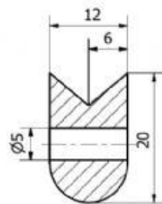
Corte G-G
