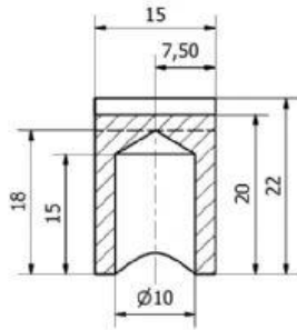
Corte G-G
