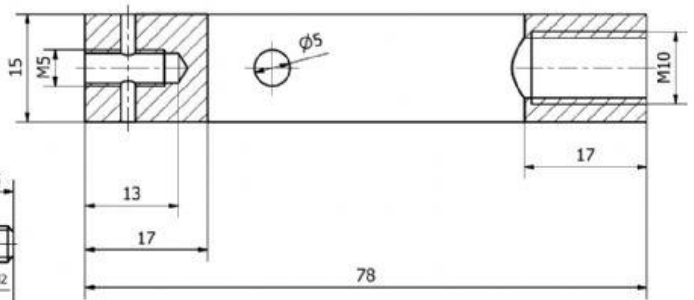
Corte E-E
