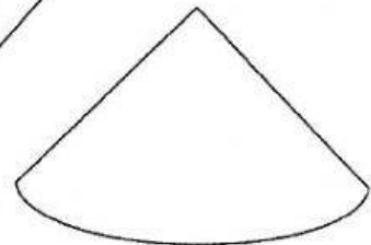
cono
