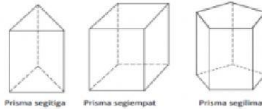
Prisma segitiga
