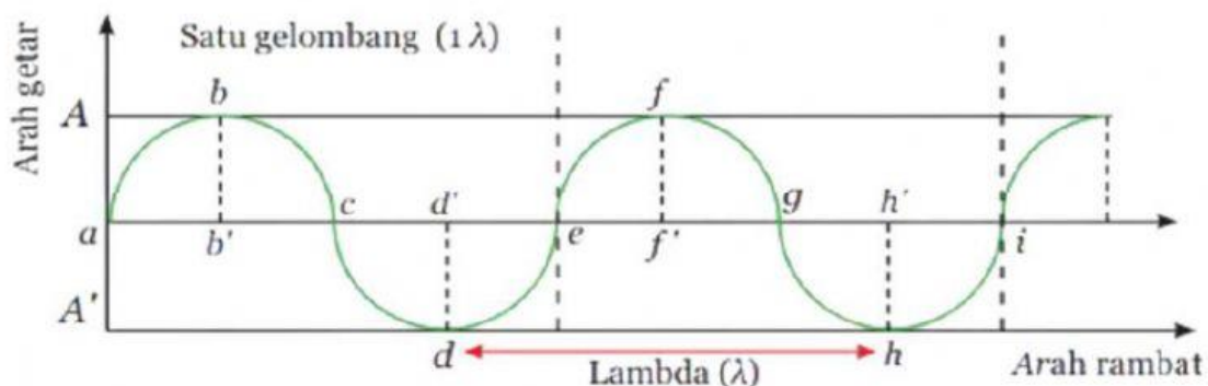
Sumber : Dok. Kemendikbud Gambar 1. Gelombang Transversal
