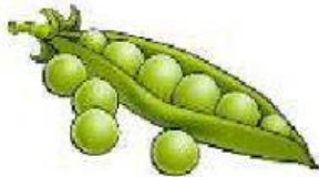
peas
