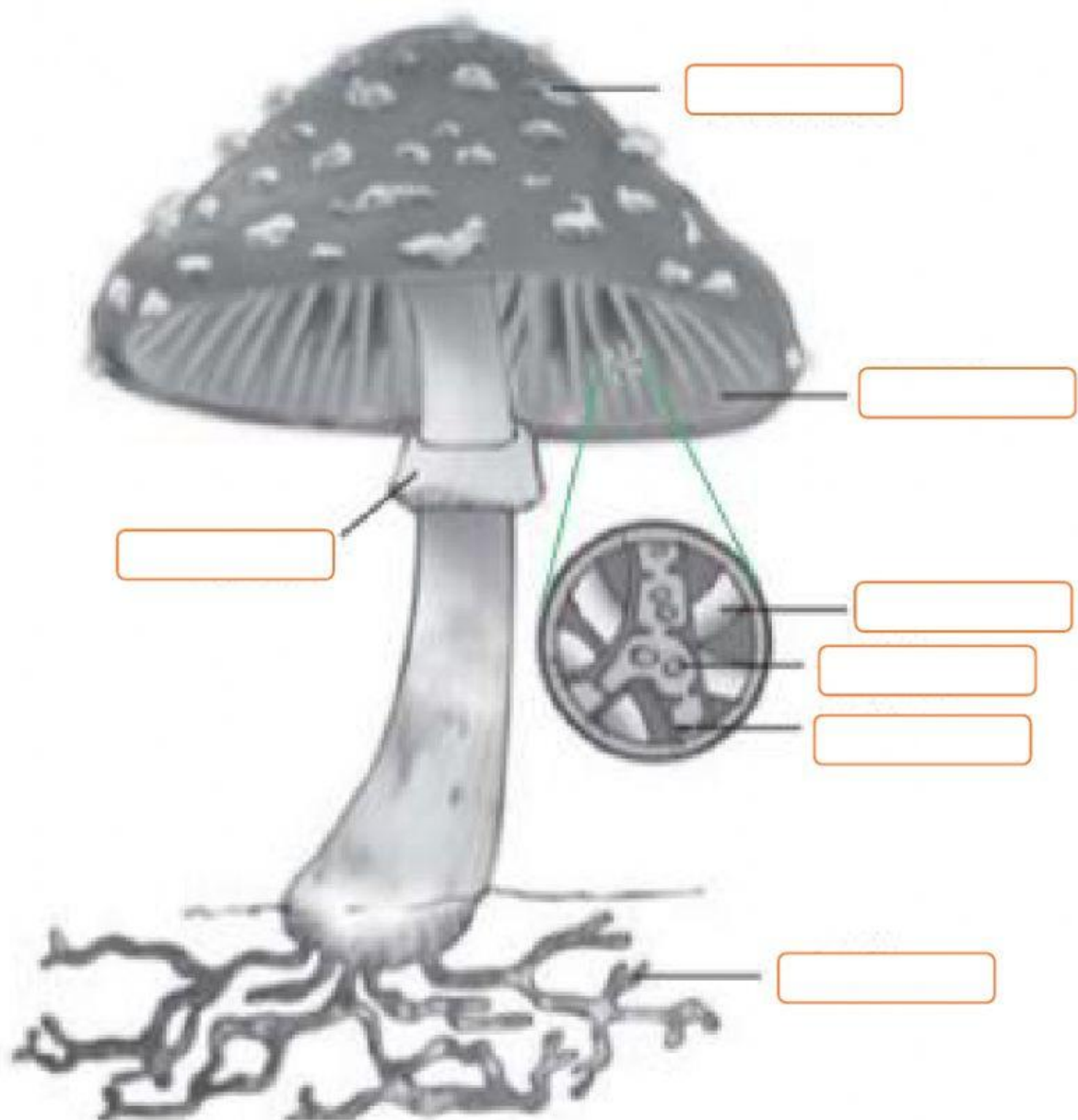
Struktur jamur
