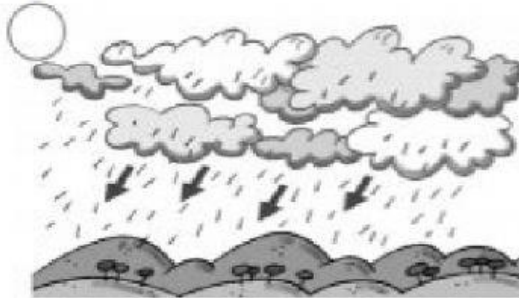
El agua de las nubes cae en forma de lluvia, nieve o granizo.
