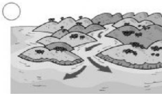
El agua vuelve al mar.
