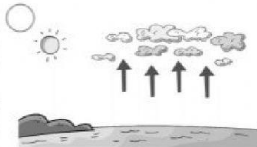
Se forman las nubes.
