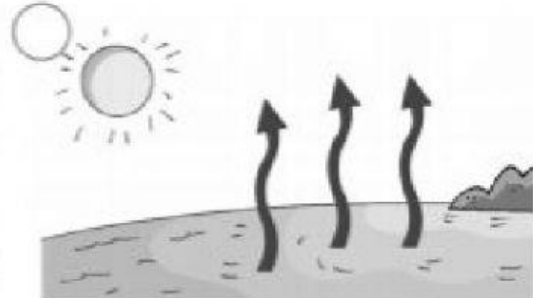
El calor del sol evapora el agua del mar.
