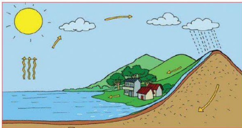
PROSES TERJADINYA HUJAN
