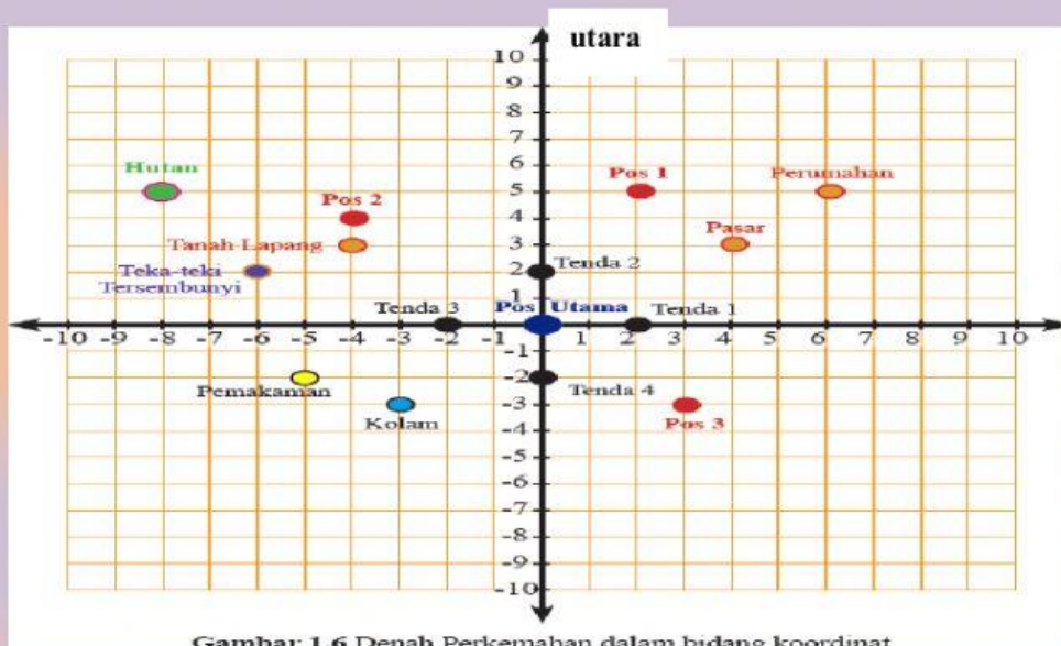
Gambar 1.6 Denah Perkemahan dalam bidang koordinat
