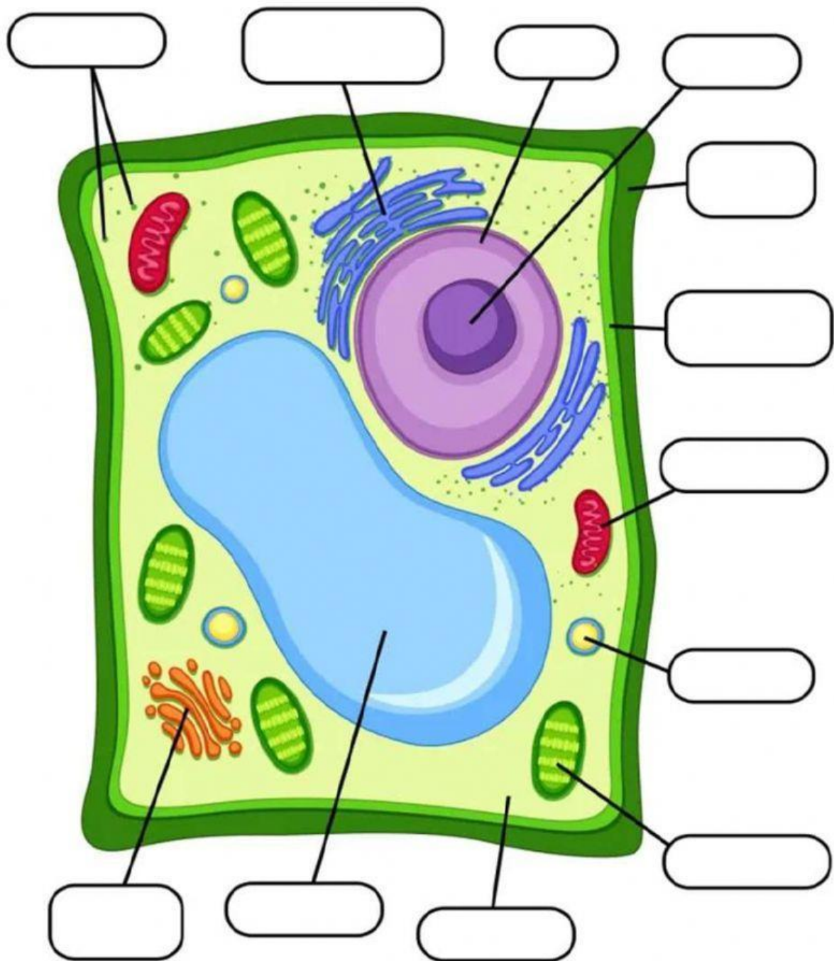
CÉLULA VEGETAL
