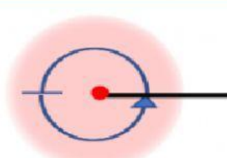
ÁNGULO COMPLETO
