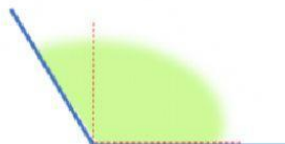
ÁNGULO OBTUSO
