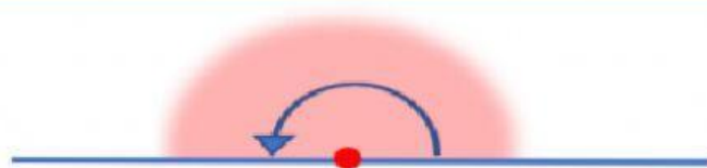
ÁNGULO LLANO
