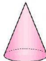
Cono
