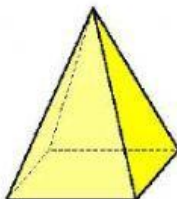
Pirámide
