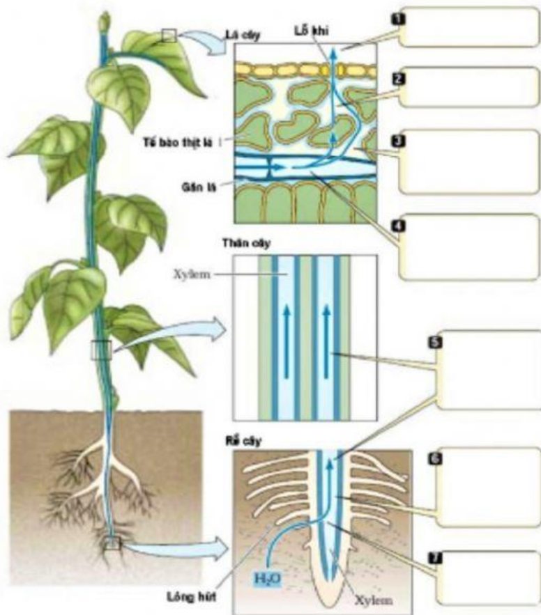
Sơ đồ vận chuyển nước từ rễ lên lá
