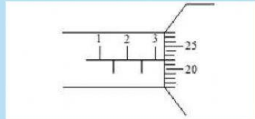
Mikrometer Sekerup
