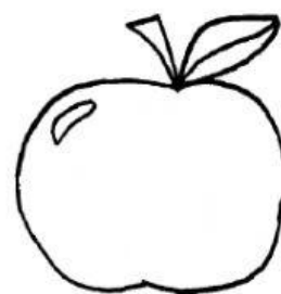
MANZANA
