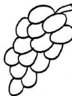
UVAS
