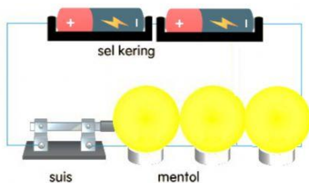
Litar Y
