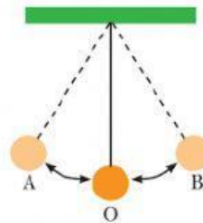
Gambar 1; Bandul Sederhana
