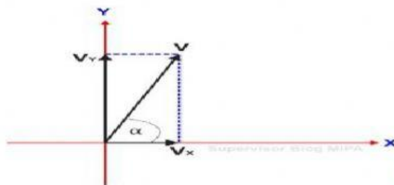
Gambar 1. Penguraian vektor
