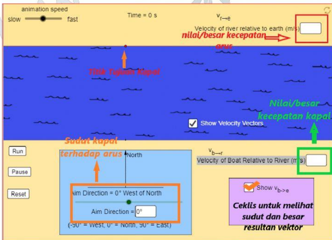
Gambar 3. Rancangan aplikasi
