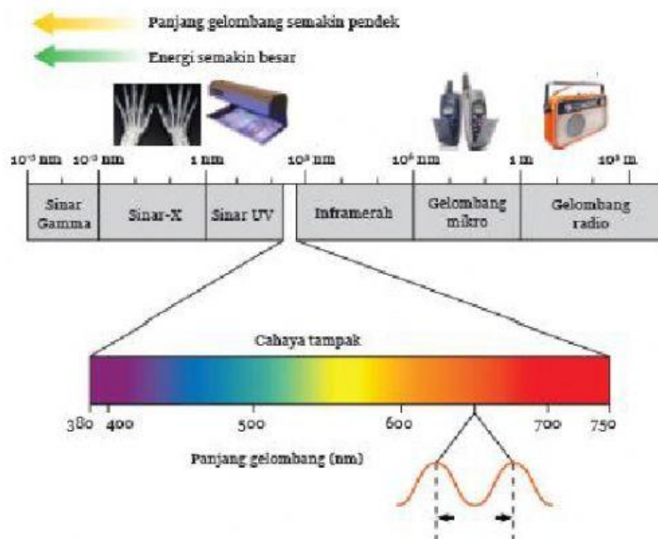
Gambar 11.8 Spektrum Elektromagnetik
