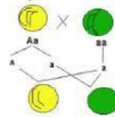
Heterocigoto
