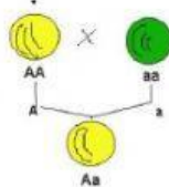
Homocigoto
