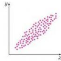
<산점도1>
