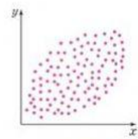
<산점도2>
