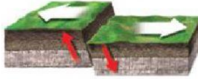
الصدع المعكوس
