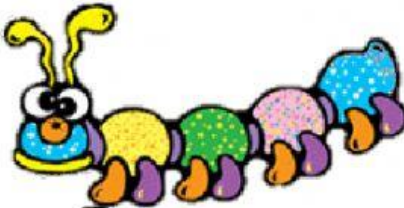
Worm 2
