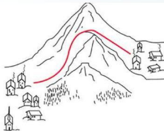
Gambar 8. Analogi energi aktivasi Sumber: Petrucci dkk. (2017, hlm. 945)
