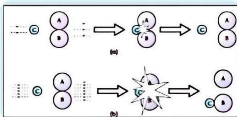
Gambar 7. (a) Energi tidak cukup untuk menghasilkan reaksi dan (b) Energi cukup untuk menghasilkan reaksi
