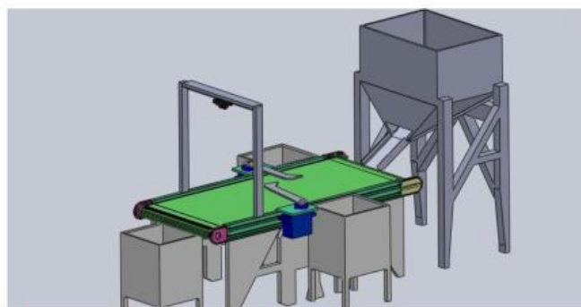
Gambar 3 Desain Sistem Konveyor Pinang (Sumber: Penulis, 2026)
