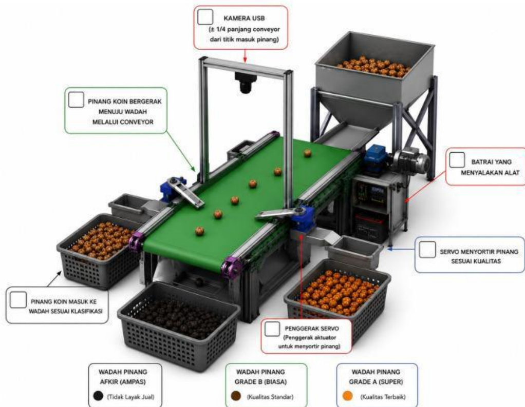
Gambar 1 Rancangan Sistem Konveyor Pinang (Sumber: ChatGPT)
