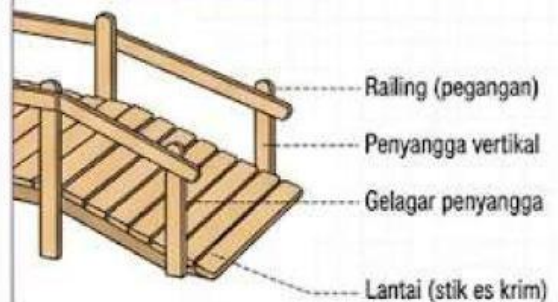
DETAIL STRUKTUR
