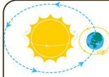
Revolusi Bumi
