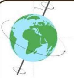
Rotasi Bumi
