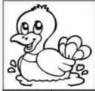
duck | ant
