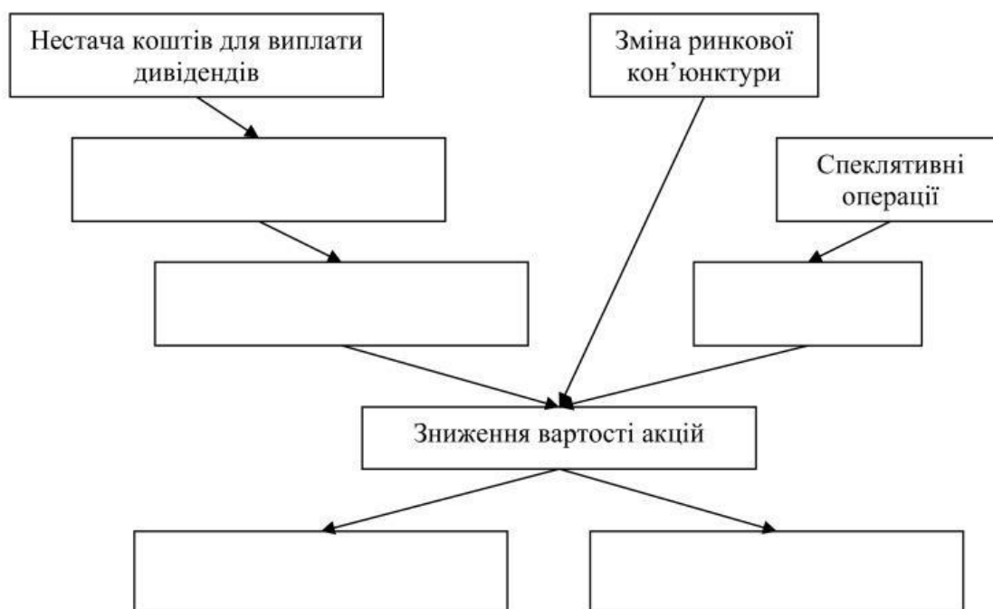
Рисунок 1 – Вихідний граф-проблем
