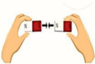
H1. Hút nhau của 2 nam châm
