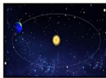
H7. Trái đất quay quanh Mặt trời
